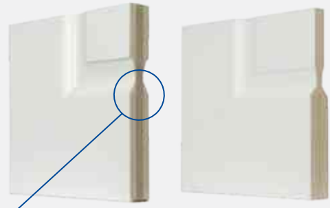
60-MINUTE FIRE DOOR
